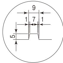
滑り止めゴム凸詳細
